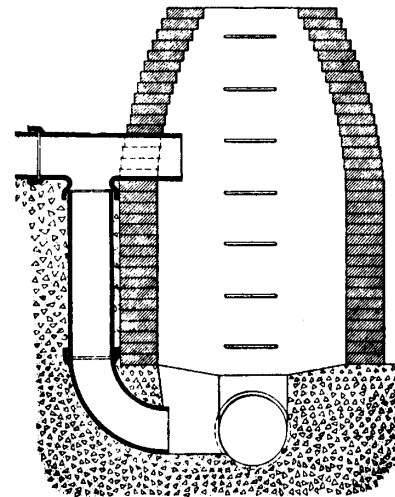
Drop Manhole
